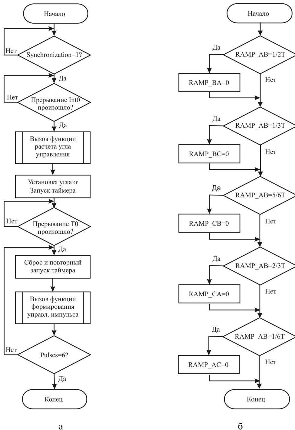
Рис. 2. Блок-схемы алгоритмов: а – формирование импульсов; б – функция формирования импульсов
