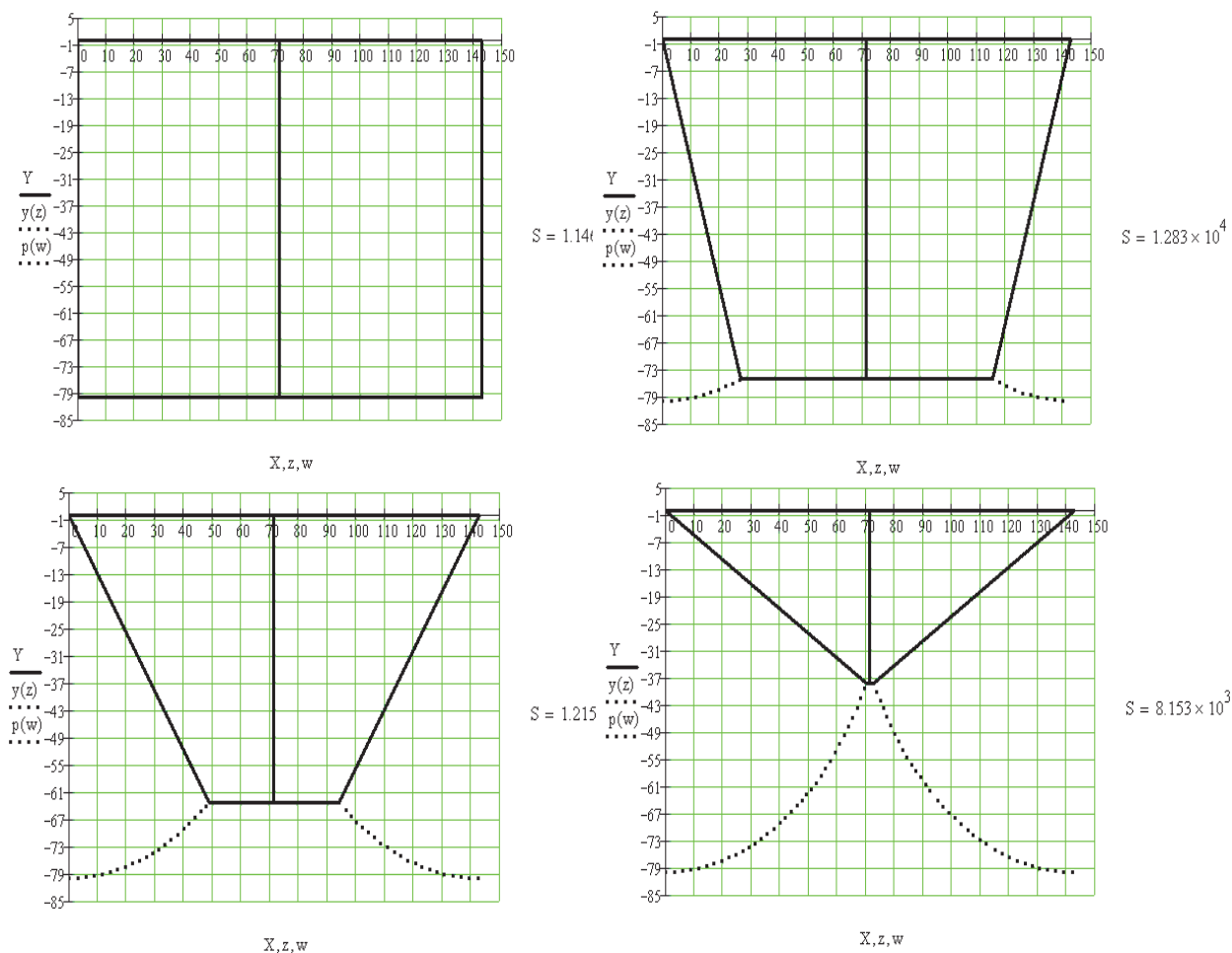
Рис. 1. Модель изменения формы кошелькового невода
