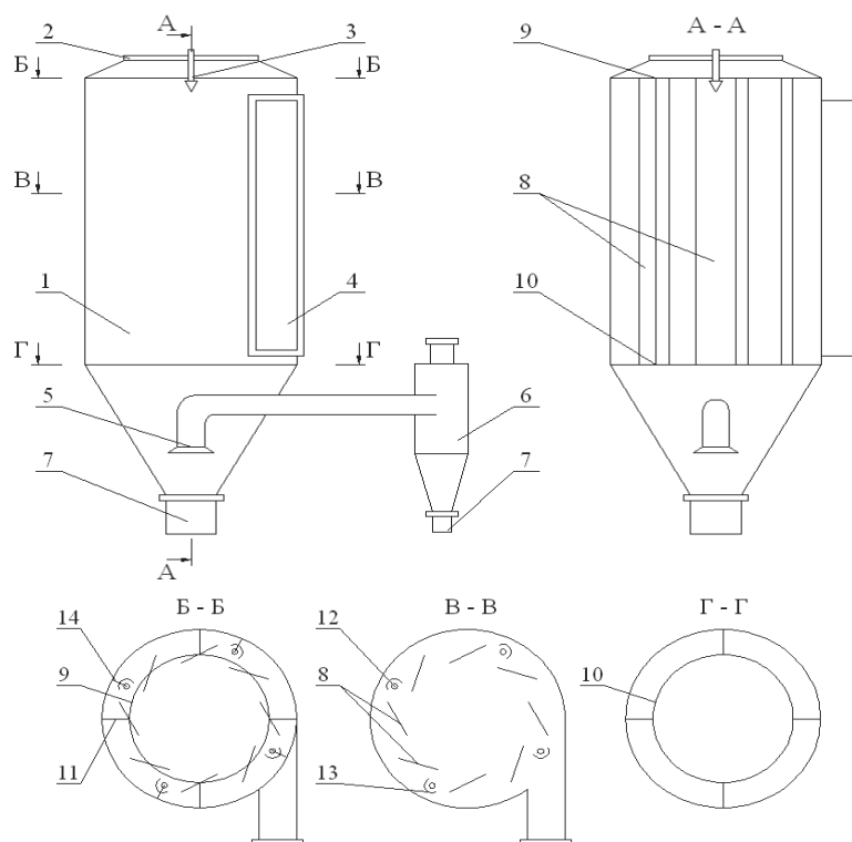
Рис. 3. Установка конвективно-радиационной распылительной суши: 1 – сушильная камера; 2, 4 – патрубок для ввода сушильного агента; 3 – распылитель; 5 – система отсоса; 6 – циклон; 7 – сборник сухого материала; 8 – вертикальные прямоугольные перегородки; 9, 10 – крепления; 11 – стержневые крепежные элементы; 12 – излучатели КГТ-220-1000; 13 – отражатели; 14 – крепления
