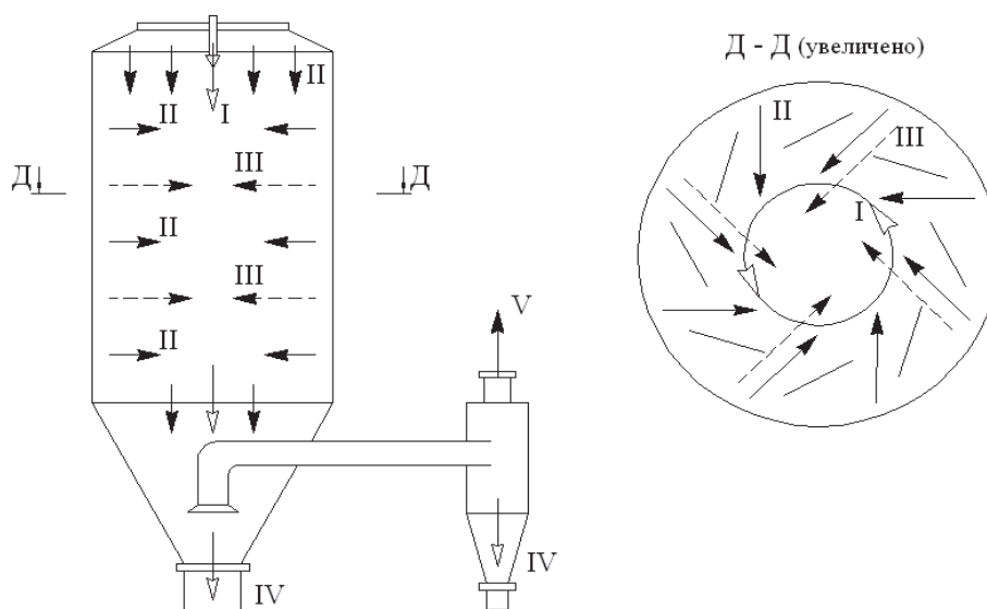
Рис. 4. Схема распределения потоков в установке конвективно-радиационной распылительной суши: I – исходный продукт; II – сушильный агент; III – инфракрасное излучение; IV – сухой продукт; V – отработавший сушильный агент
