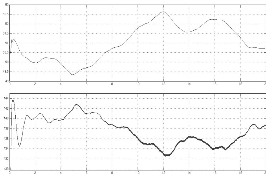
Рис. 2. Осциллограммы изменения частоты напряжения генератора и выходного напряжения полупроводникового преобразователя
