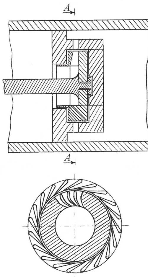
Рис. 4. Схема радиальной турбины с частичным облопачиванием рабочего колеса
