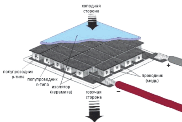
Рис. 1. Термоэлектрический модуль
