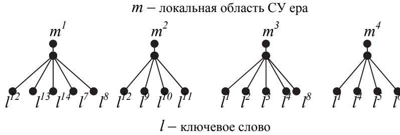
Рис. 2. Двудольный граф предиката P_l(l,m)
